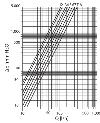
R401PTG-R402PTG
