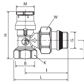
R401PTG
