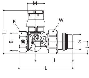
R402TG
