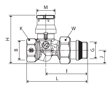
R402PTG
